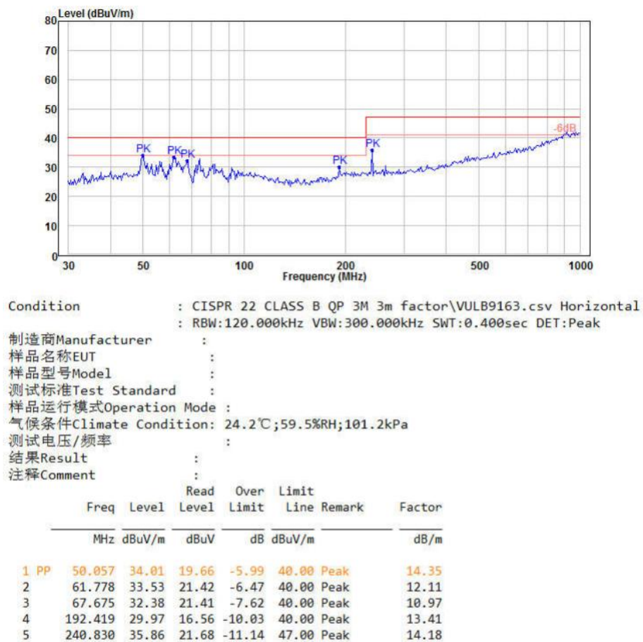
图 5-7 辐射测试垂直方向
