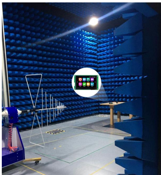
图 5-5 辐射测试图
