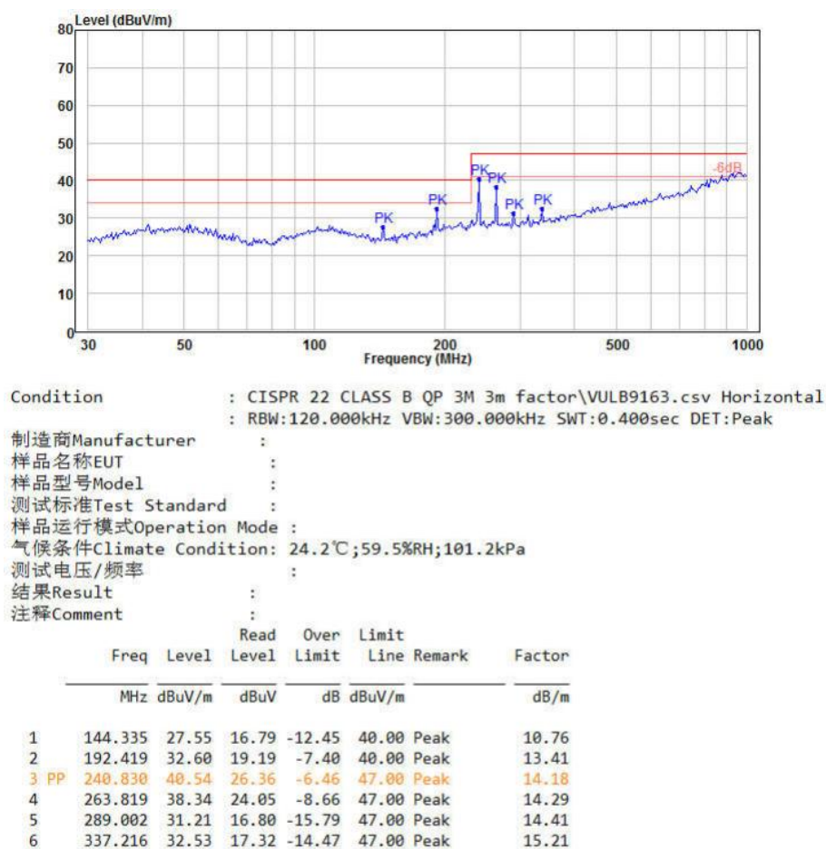
图 5-6 辐射测试水平方向
