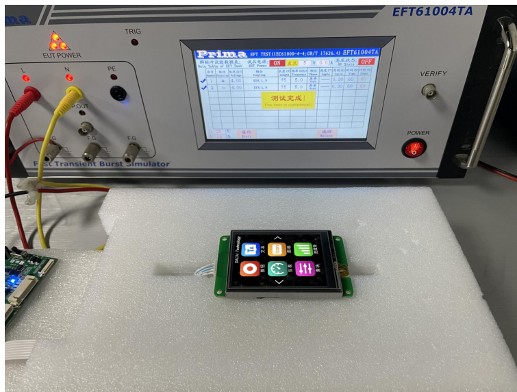
图 5-4 群脉冲测试图
