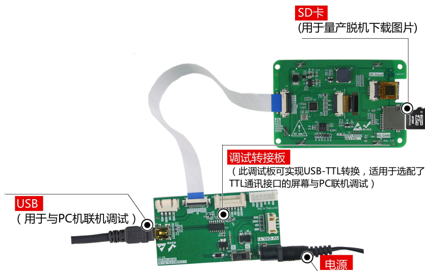
图 1-5 调试工具图
