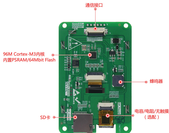
图 1-4 硬件配置图
